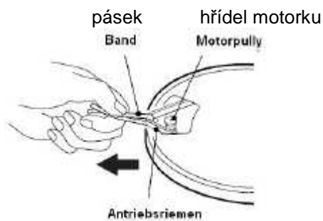
řemínek pohonu
