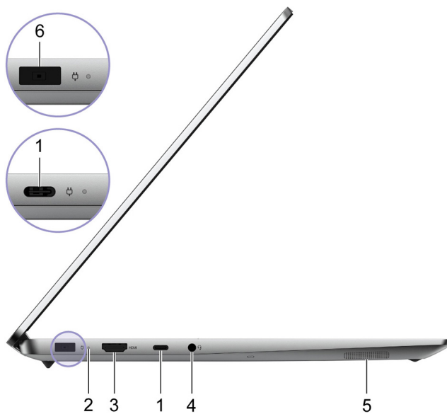
Obrázok 5. IdeaPad 5 Pro 14ARH7 a IdeaPad 5 Pro 14IAP7
