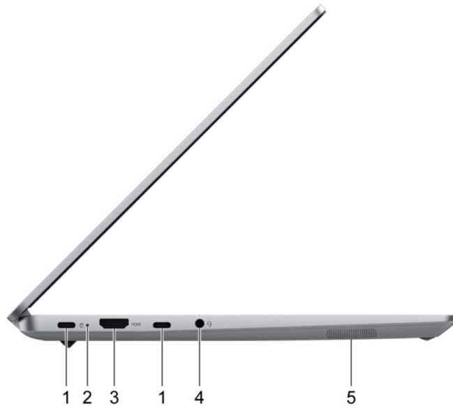
Obrázok 5. IdeaPad 5 Pro 14ARH7 a IdeaPad 5 Pro 14IAP7
