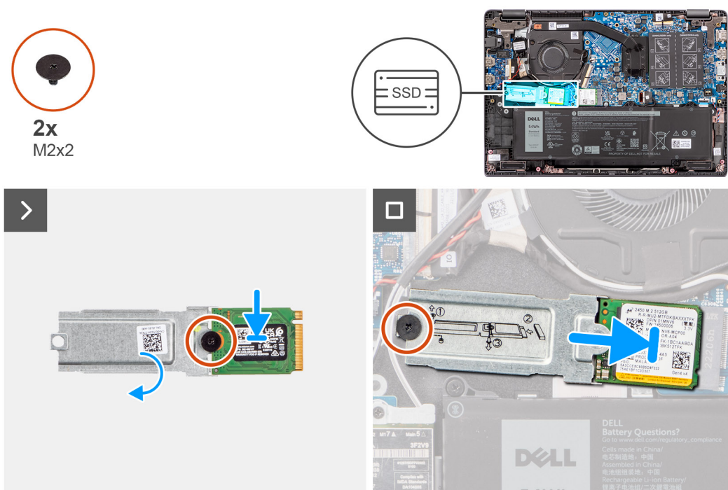
Obrázok 23. Montáž disku SSD M.2 2230
