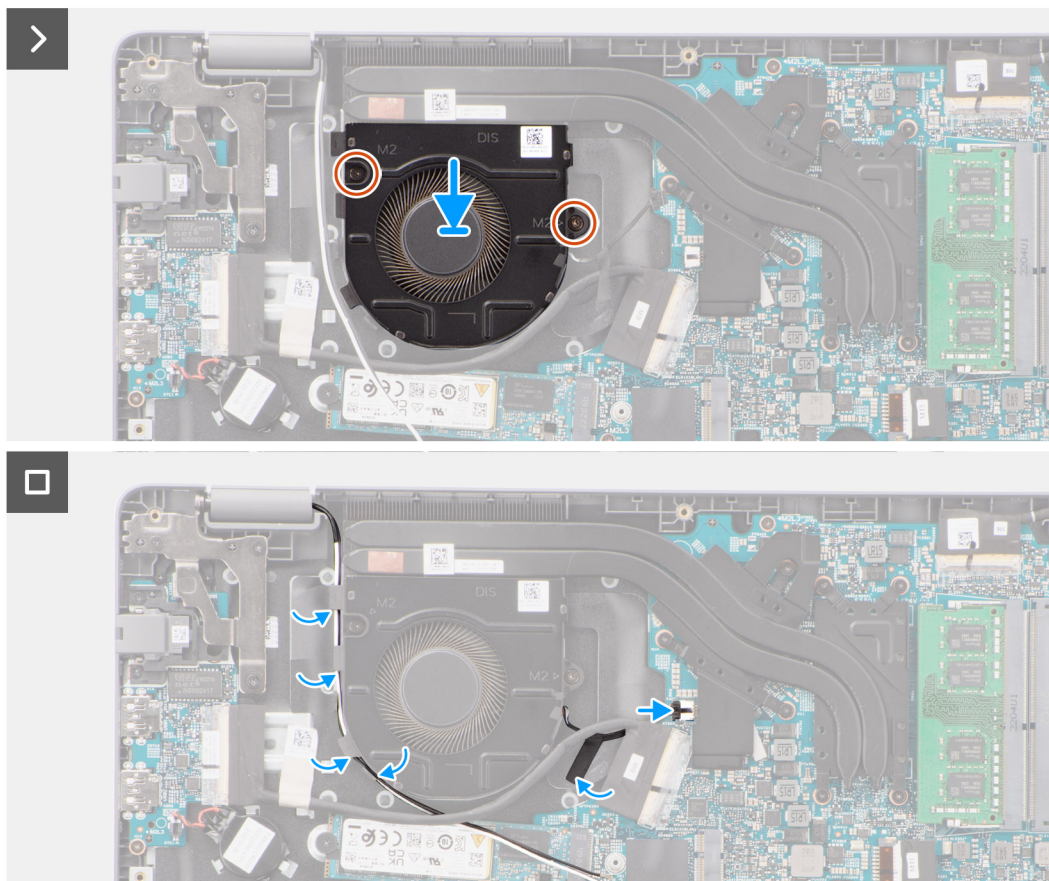
Obrázok 34. Montáž ventilátora
