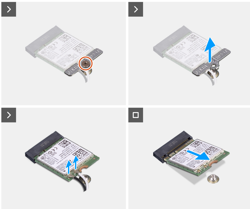
Obrázok 14. Demontáž karty bezdrôtovej komunikácie
