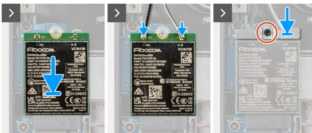
Obrázok 17. Montáž karty WWAN
