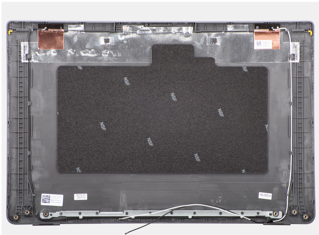
Obrázok 70. Demontáž zadného krytu obrazovky
