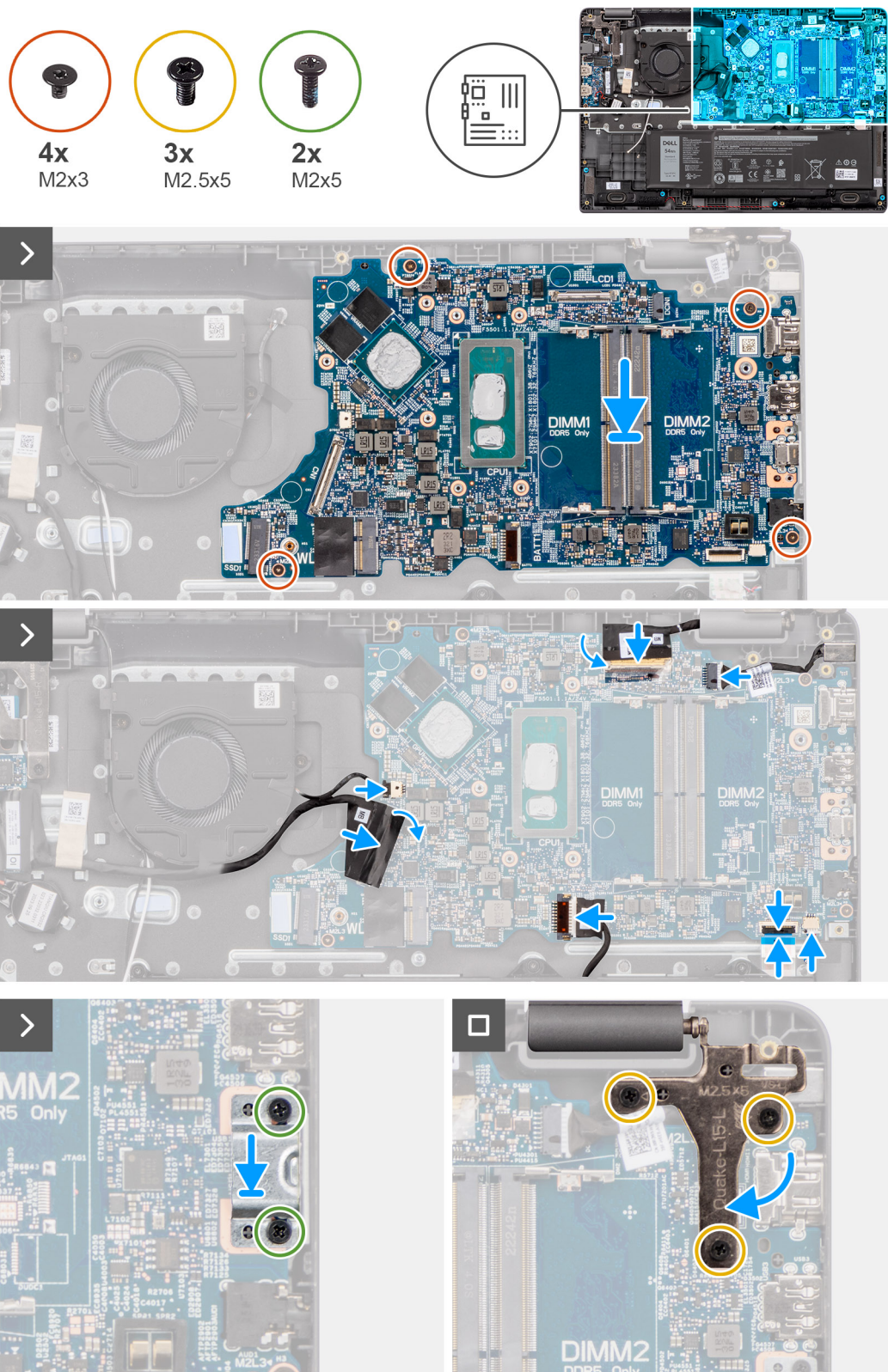
Obrázok 45. Montáž systémovej dosky
