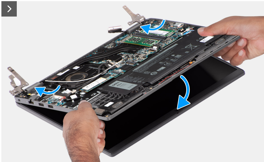
Obrázok 51. Montáž zostavy obrazovky
