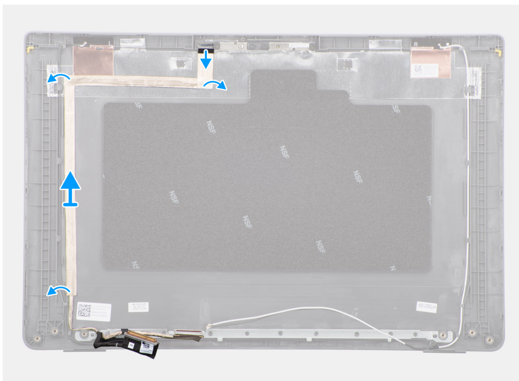
Obrázok 68. Demontáž kábla eDP
