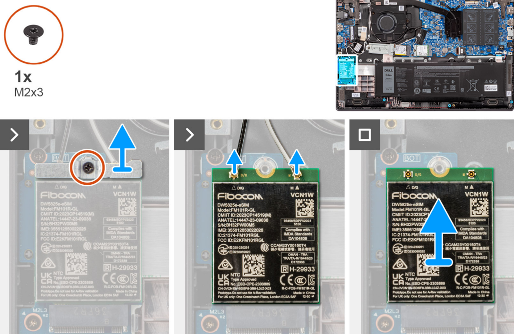
Obrázok 16. Demontáž karty WWAN
