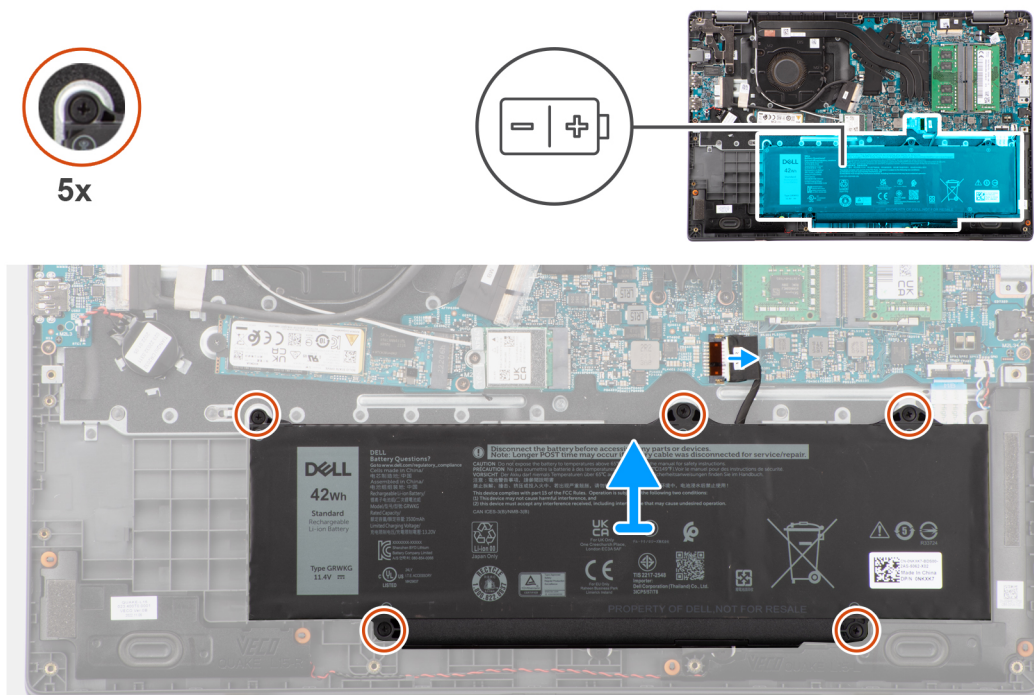
Obrázok 24. Demontáž batérie
