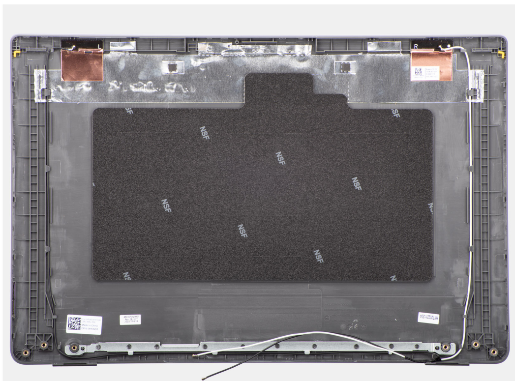
Obrázok 71. Montáž zadného krytu obrazovky
