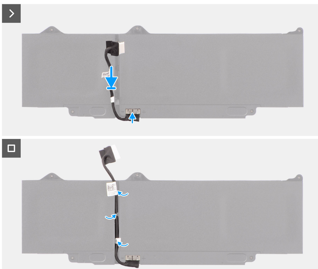
Obrázok 26. Pripojenie kábla batérie
