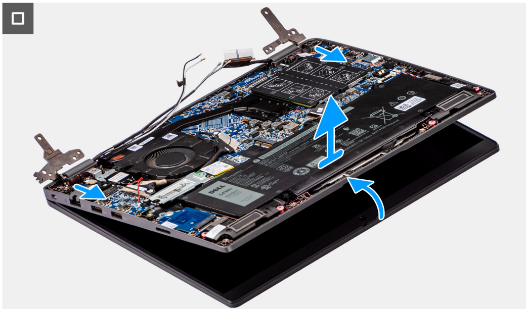
Obrázok 49. Demontáž zostavy obrazovky
