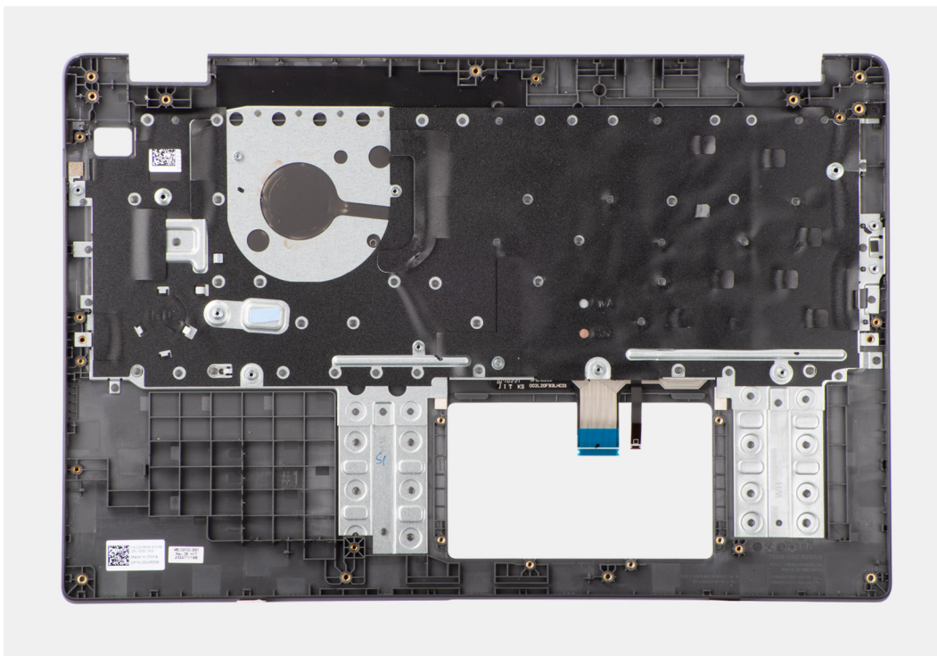
Obrázok 46. Demontáž zostavy opierky dlaní a klávesnice
