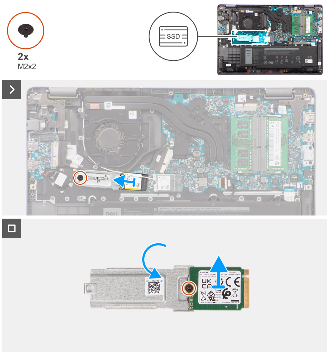
Obrázok 22. Demontáž disku SSD M.2 2230
