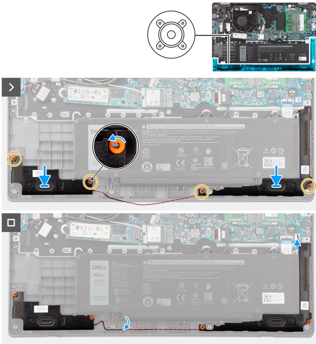
Obrázok 21. Montáž reproduktorov
