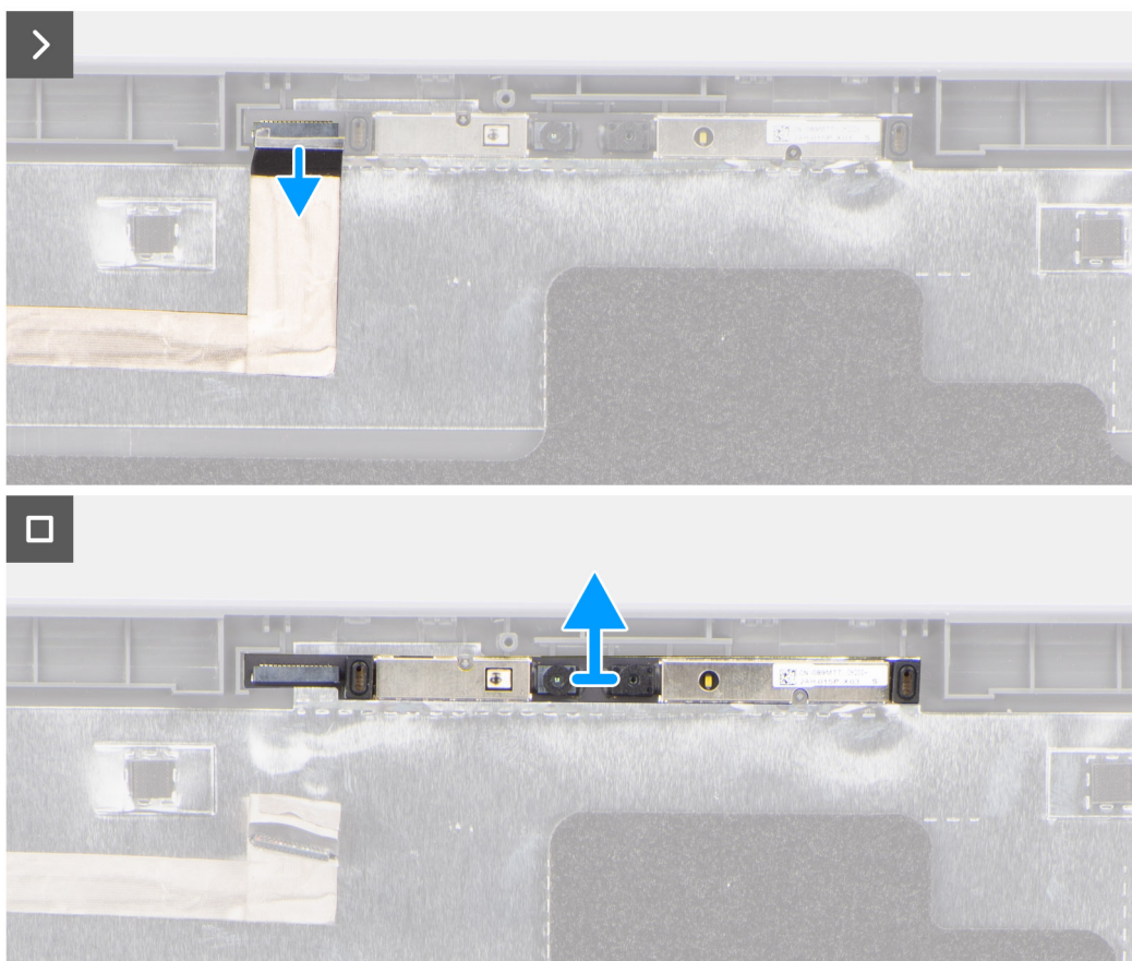
Obrázok 66. Demontáž kamery
