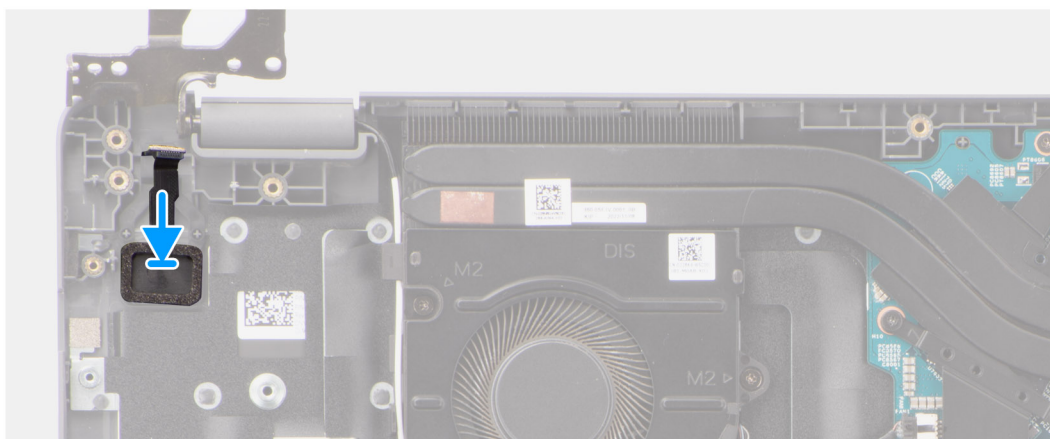
Obrázok 40. Montáž tlačidla napájania
