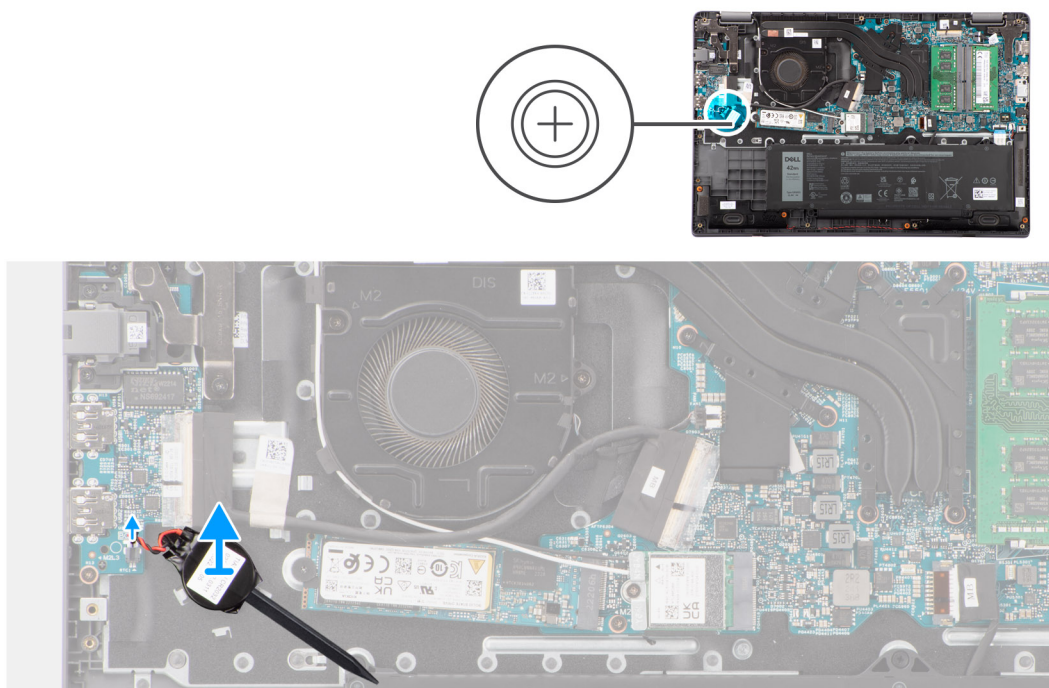
Obrázok 18. Demontáž gombíkovej batérie
