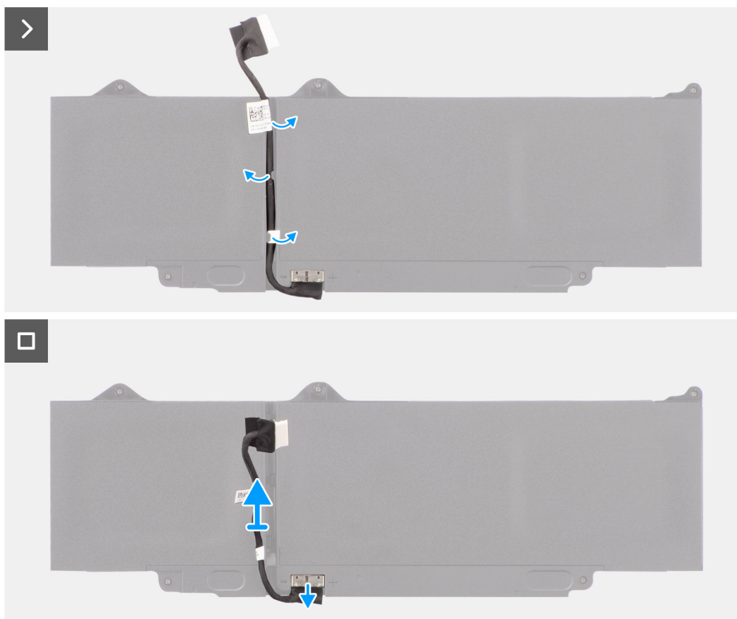
Obrázok 25. Demontáž kábla batérie
