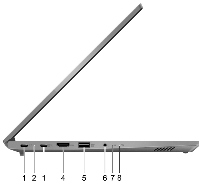
Obrázok 5. Pohľad z ľavej strany—ThinkBook 14 G2 ARE a ThinkBook 15 G2 ARE
