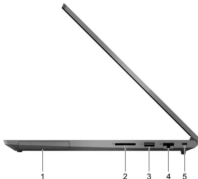
Obrázok 7. Pohľad z pravej strany—ThinkBook 15 G2 ITL a ThinkBook 15 G2 ARE
